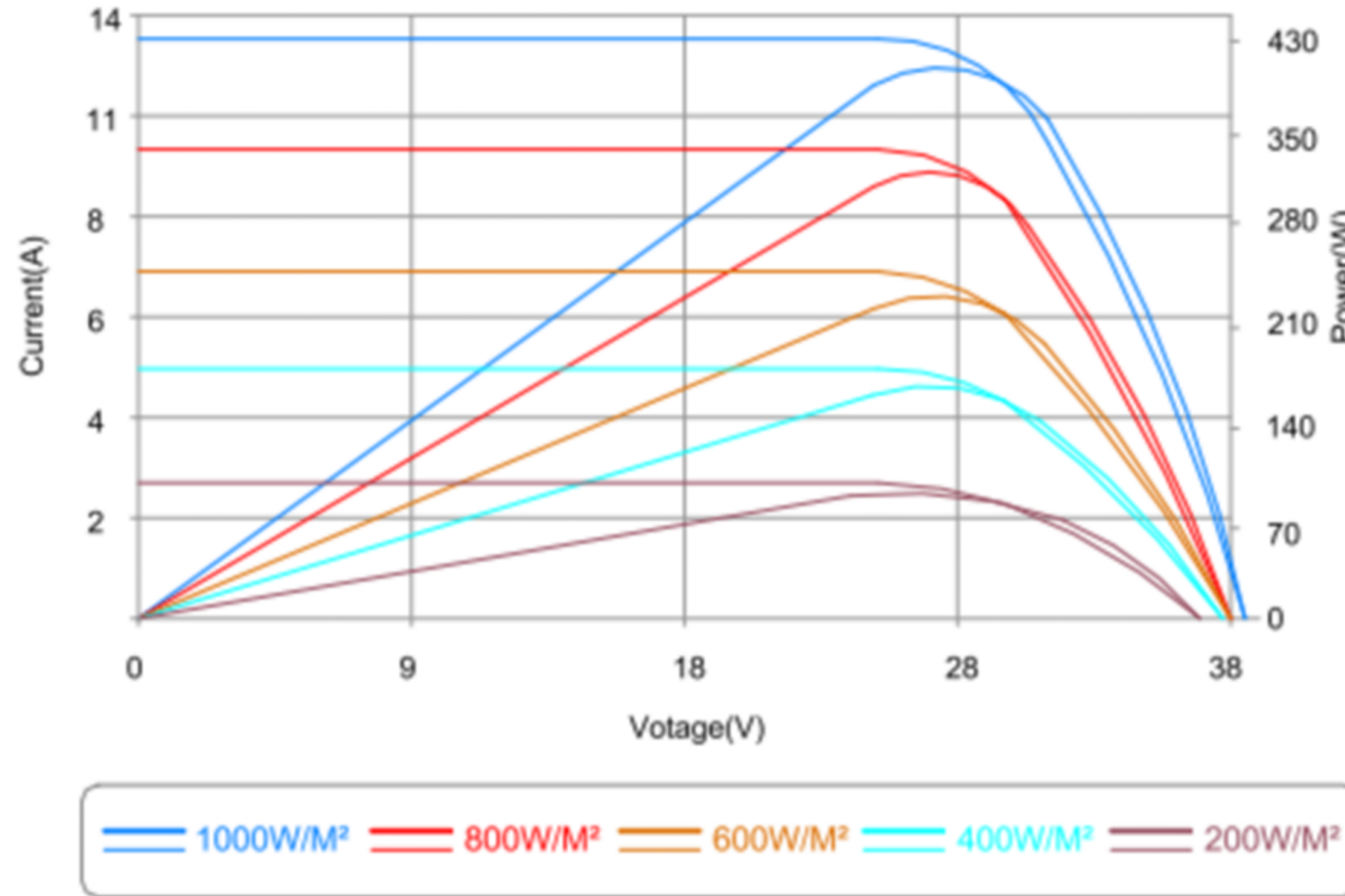
电流-电压& 功率-电压曲线图 (410W) Currnt-Voltage&Power-Voltage Curve
