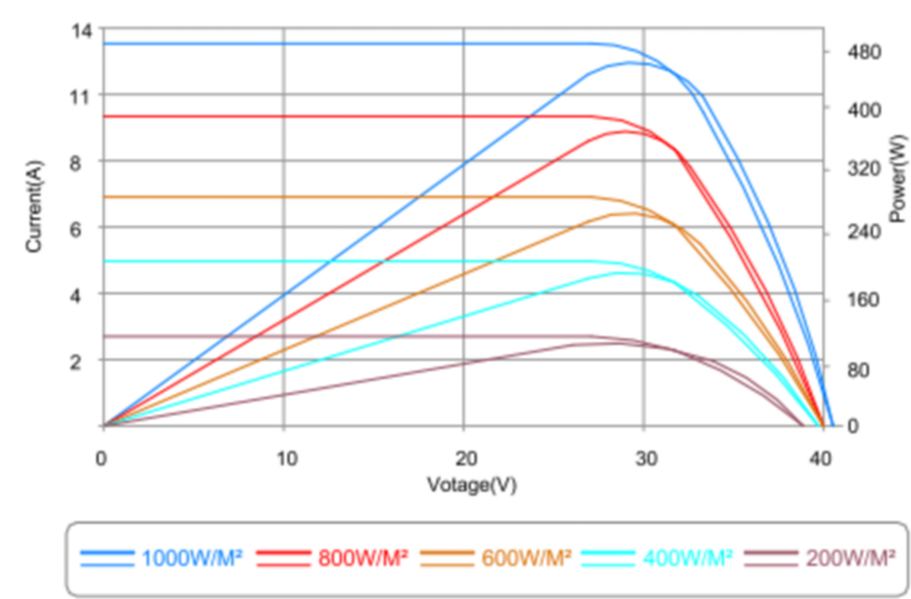
电流-电压& 功率-电压曲线图（450w） Currt-Voltage&Power-Voltage Curve
